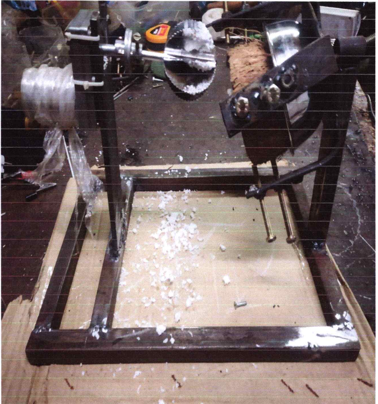
MINI COCONUT SCRAPING MACHINE
